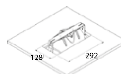
Inbouwrand plafondmodel
